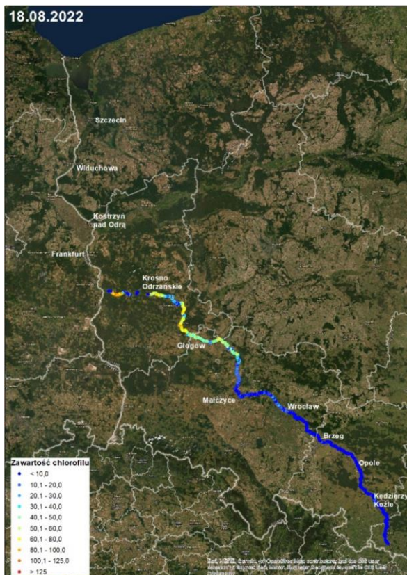
Rycina IV.9 Rozkład zawartości chlorofilu w wodach Odry w okresie 18.08.2022 oraz 25-26.08.2022 opracowany na podstawie zdjęć satelitarnych Sentinel-2
