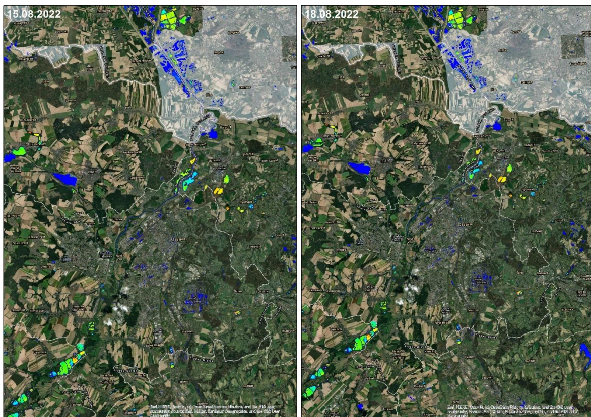
Rycina IV.12 Rozkłady chlorofilu w górnym biegu rzeki Odry na odcinku Ostrava – Chałupki w dniach 15 i 18 sierpnia 2022 r. opracowane na podstawie zdjęć satelitarnych Sentinel-2
