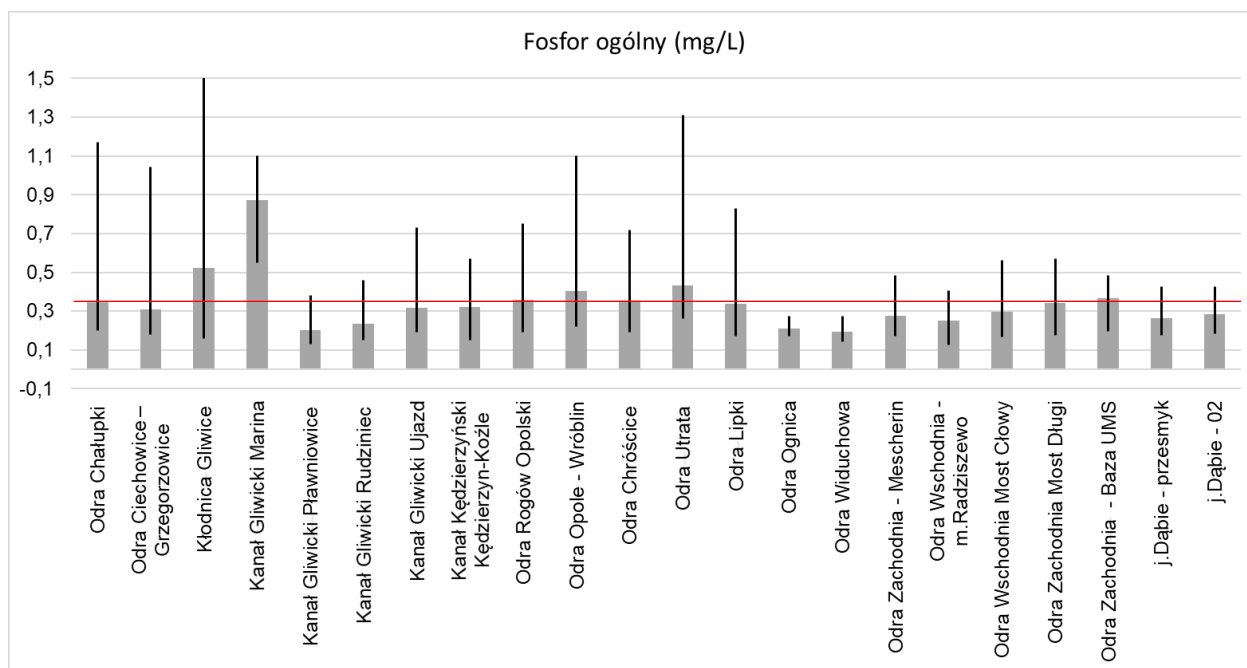
Rycina III.16 Zmiany stężenia fosforu ogólnego (mg/L) na stanowiskach monitorowanych przez Centralne Laboratorium Badawcze GIOŚ w okresie 28.07 – 20.09. br. Czerwona linia orientacyjnie wyznacza wartość graniczną stanu dobrego dla wielkich rzek nizinnych (0,35 mg/L)
