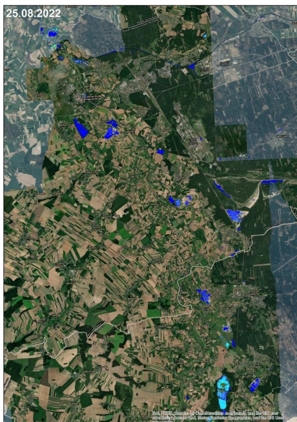
Rycina IV.16 Rozkłady chlorofilu w górnym biegu rzeki Odry na odcinku Racibórz – Śluza Januszkowice w dniu 18 i 25 sierpnia 2022 r. opracowane na podstawie zdjęć satelitarnych Sentinel-2
