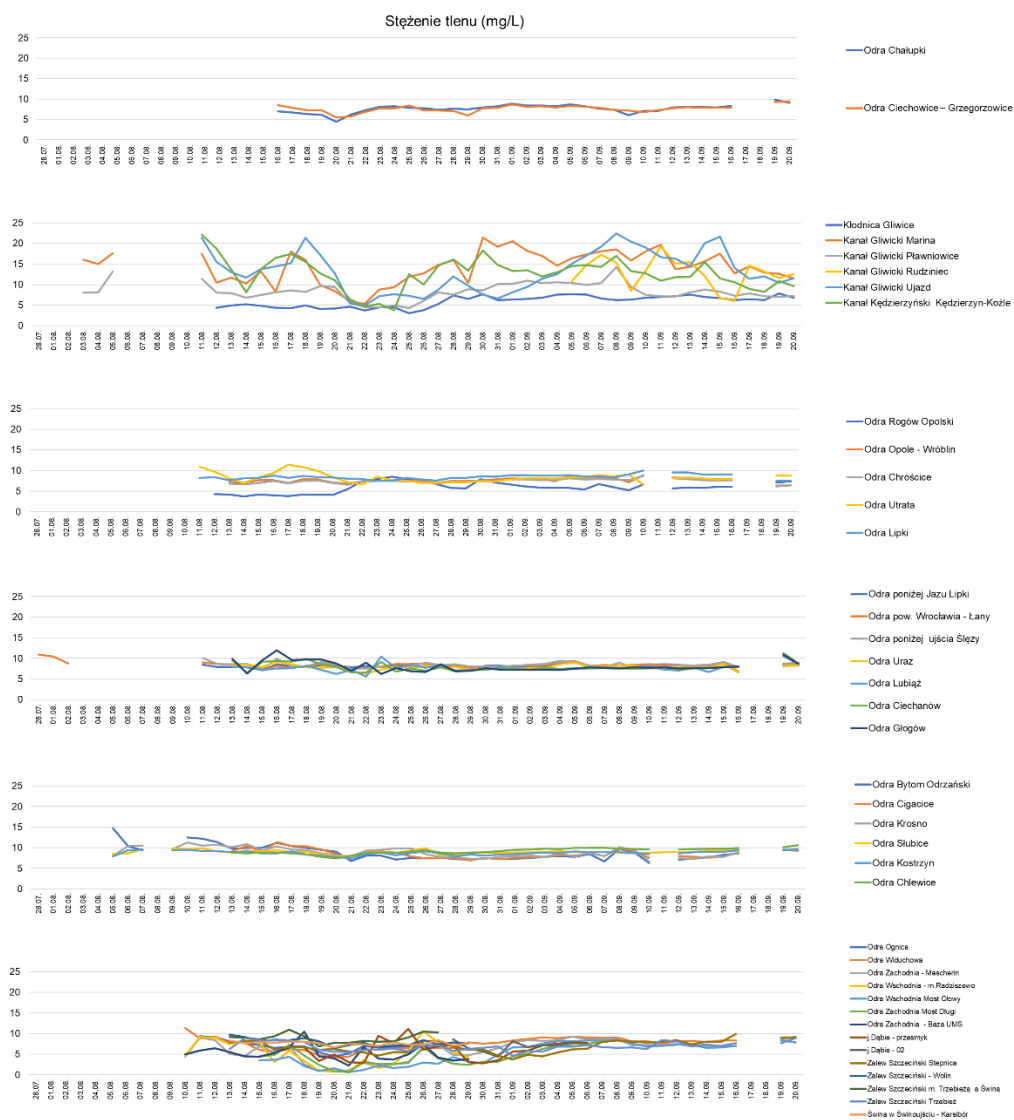
Ryc. III.12 Zmiany stężenia tlenu w wodach na stanowiskach monitorowanych przez Centralne Laboratorium Badawcze GIOŚ w okresie 28.07 – 20.09. br. z uwzględnieniem granic administracyjnych województw i typu ciek (W kolejności od góry: śląskie, śląskie/opolskie – kanały, opolskie, dolnośląskie, lubuskie, zachodniopomorskie).
