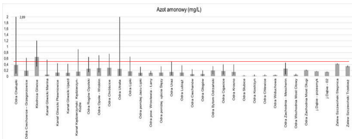
Rycina III.15 Zmiany stężenia azotu amonowego (mg/L) na stanowiskach monitorowanych przez Centralne Laboratorium Badawcze GIOŚ w okresie 28.07 – 20.09. br. Czerwona linia orientacyjnie wyznacza wartość graniczną stanu dobrego dla wielkich rzek nizinnych (0,45 mg/L)
