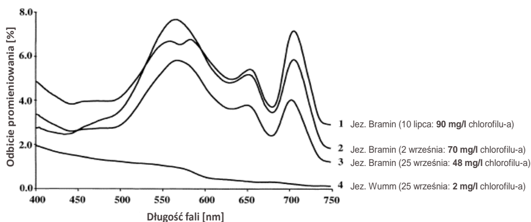
Rycina IV.2 Wpływ zawartości chlorofilu-a na właściwości odbicia promieniowania dla wód jeziornych – przykład jezior Meklemburgii (Thiemann i Kaufmann, 2002)
