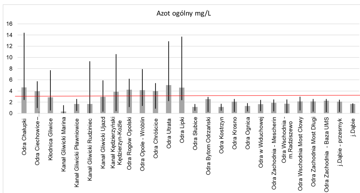
Rycina III.13 Zmiany stężenia azotu ogólnego (wartość średnia – szary słupek, minimalna, maksymalna – czarna linia) na stanowiskach monitorowanych przez Centralne Laboratorium Badawcze GIOŚ w okresie 28.07 – 20.09. br. Czerwona linia orientacyjnie wyznacza wartość graniczną stanu dobrego dla wielkich rzek nizinnych (3,5 mg/L)
