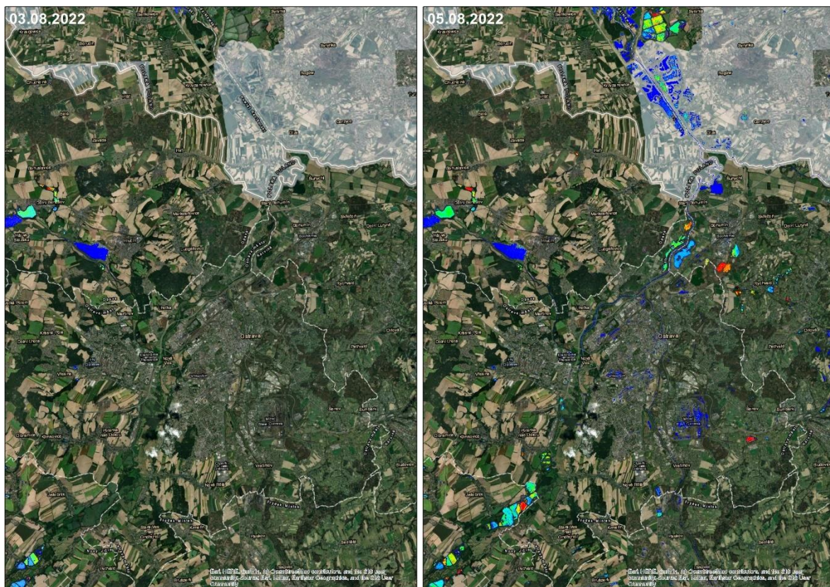
Rycina IV.11 Rozkłady chlorofilu w górnym biegu rzeki Odry na odcinku Ostrava – Chałupki w dniach 3 i 5 sierpnia 2022 r. opracowane na podstawie zdjęć satelitarnych Sentinel-2
