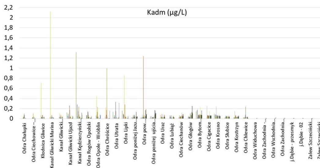
Rycina III.18 Zmiany stężenia kadmu (mg/L) na stanowiskach monitorowanych przez Centralne Laboratorium Badawcze GIOŚ w okresie 28.07 – 20.09. br.
