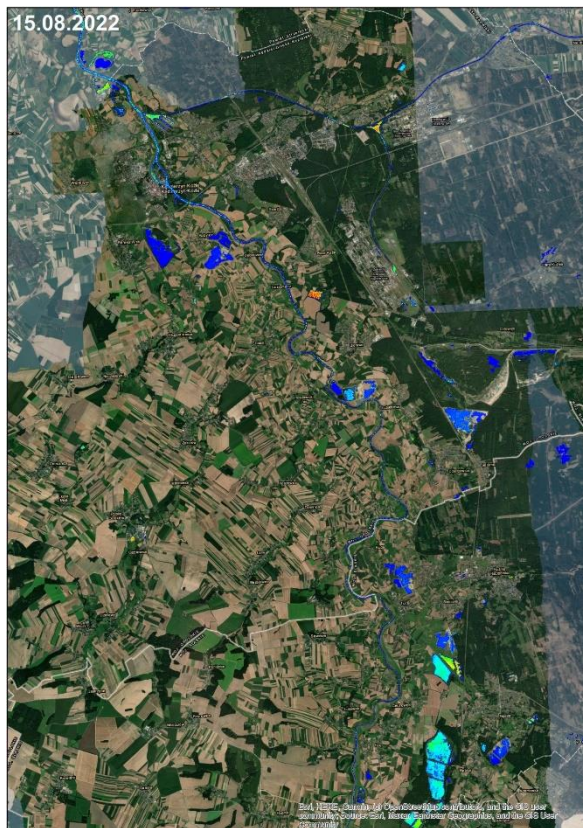
Rycina IV.15 Rozkłady chlorofilu w górnym biegu rzeki Odry na odcinku Racibórz – Śluza Januszkowice w dniach 5 i 15 sierpnia 2022 r. opracowane na podstawie zdjęć satelitarnych Sentinel-2
