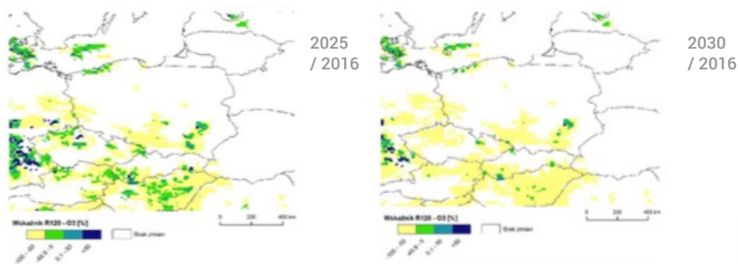
Rysunek 13. Liczba dni z przekroczeniem poziomu 120 µg/m 3 dla najwyższej ośmiogodzinnej średniej kroczącej stężeń ozonu w ciągu doby
