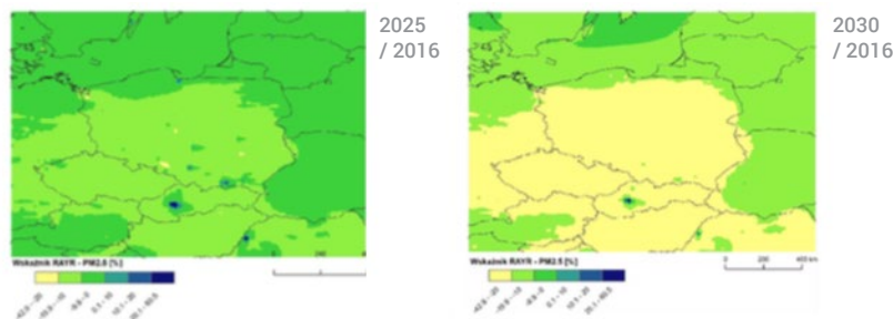
Rysunek 6. Względna zmiana stężenia średniorocznego PM 2,5 w roku 2025 (lewy panel) i 2030 (prawy panel) w stosunku do roku 2016.
